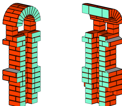
Поперечный и продольный разрезы
