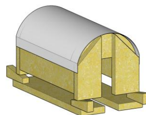
Кружало в сборе с установочным комплектом
