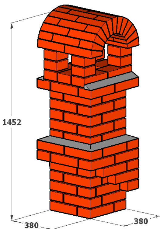
Труба в сборе
