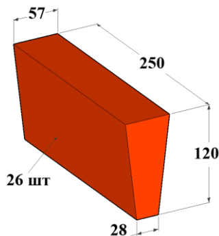
Клиновой кирпич для зонта
