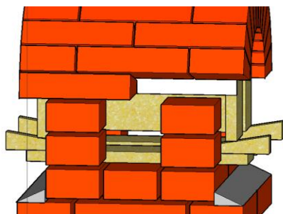
Привязка кружала к кирпичной кладке
